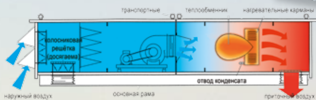
Функциональная схема
